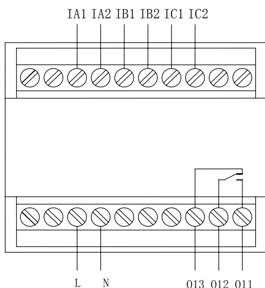
AMDS-□/A041 系列保护器主单元接线端子图
