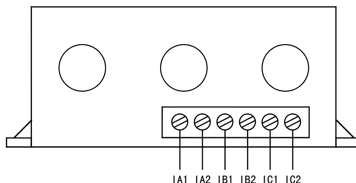
AMDS-□/A04□ 系列保护器电流检测单元接线端子图
