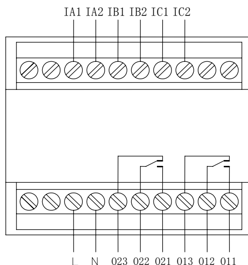
AMDS-□/A042 系列保护器主单元接线端子图
