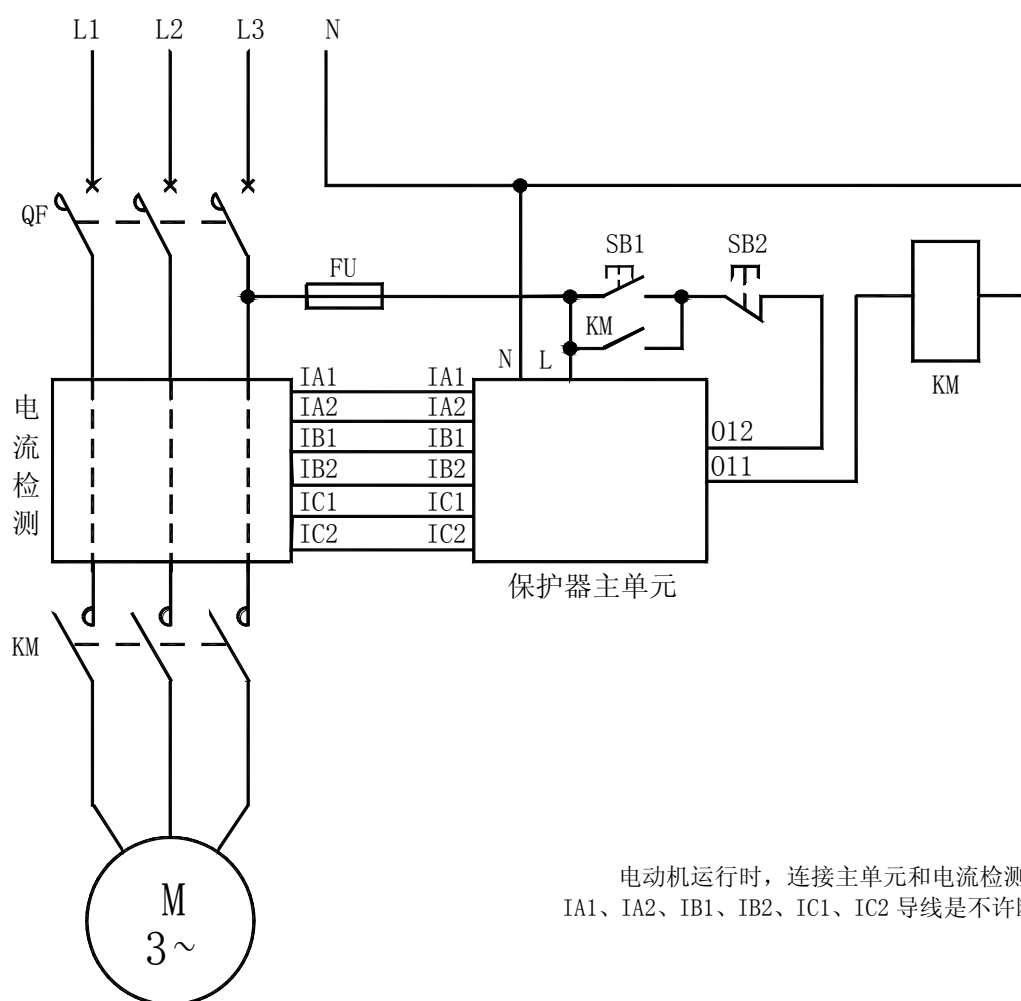
AMDS-□/A04□ 系列电动机保护器应用电气原理图
