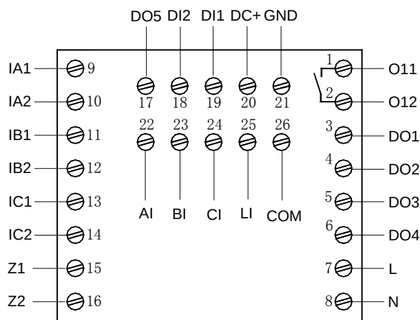
AMDPH-X/E811 系列保护器主单元接线端子图
