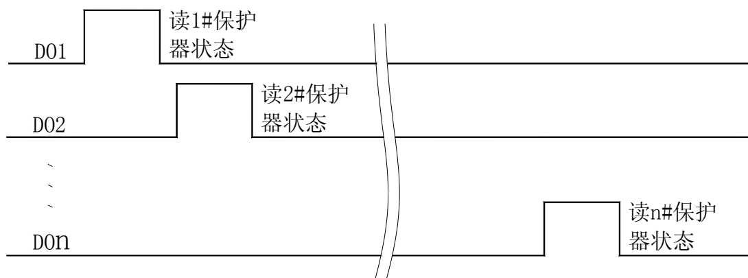
PLC 读取多台 AMDPH-X/E811 系列电动机保护器时序图
