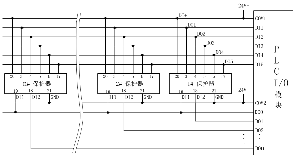
PLC 读取多台 AMDPH-X/E811 系列电动机保护器电气原理图
