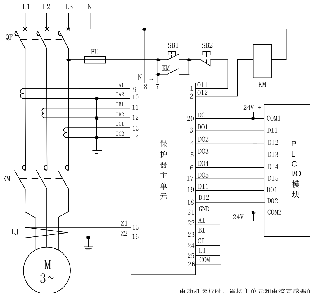
AMDPH-X/E811 系列电动机保护器 DO 连接 PLC 电气原理图
