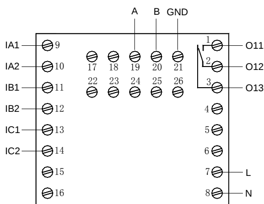
AMDPH-X/E221 系列保护器主单元接线端子图
