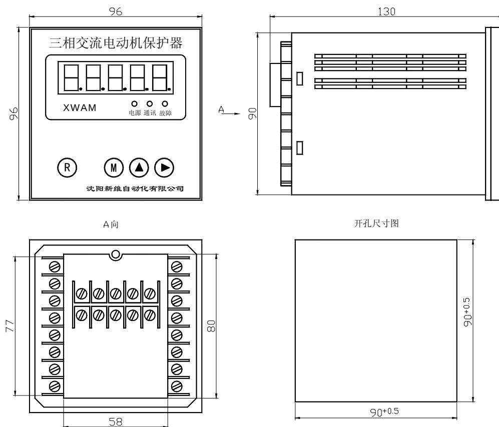
AMDPH-X/E22□ 系列电动机保护器主单元外形及安装孔尺寸
