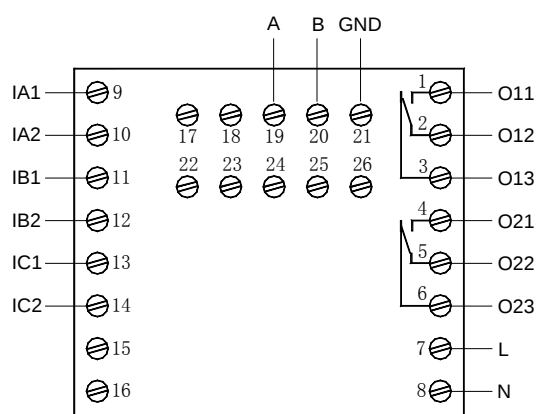
AMDPH-X/E222 系列保护器主单元接线端子图
