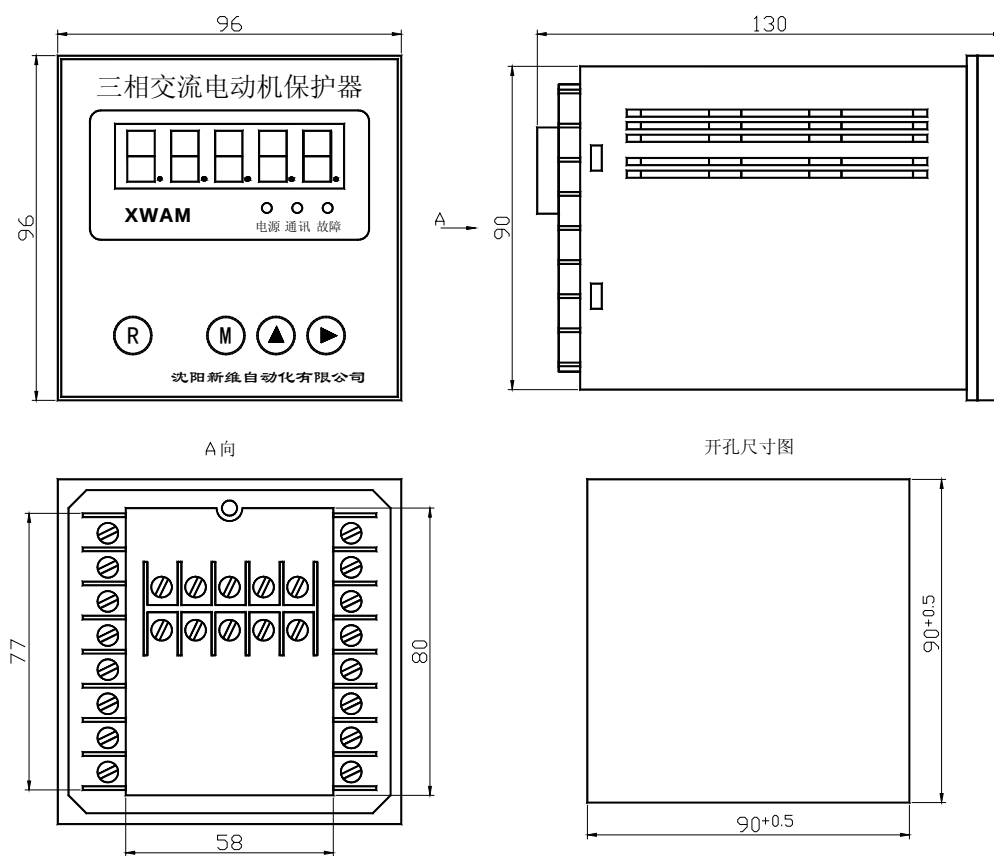
AMDPH-X/E20□ 系列电动机保护器主单元外形及安装孔尺寸
