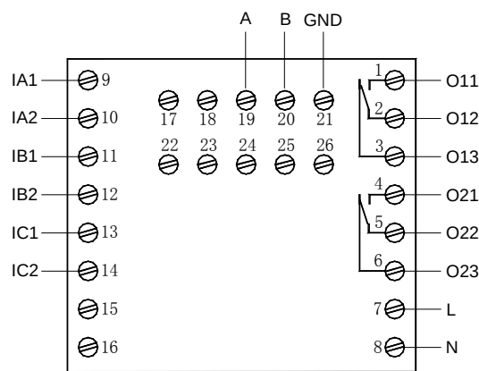
AMDPH-X/E202 系列保护器主单元接线端子图
