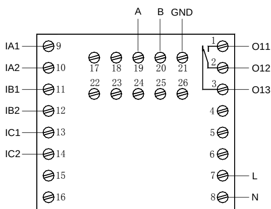
AMDPH-X/E201 系列保护器主单元接线端子图
