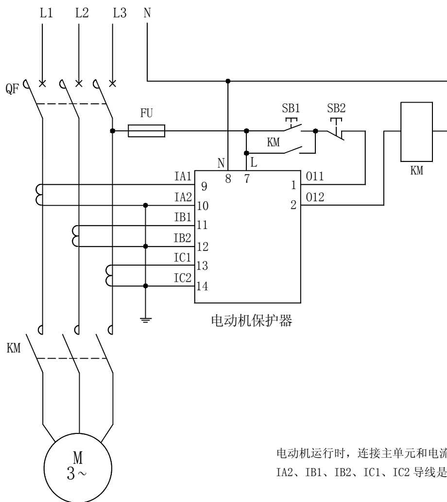
AMDPH-X/E00□ 系列电动机保护器应用电气原理图
