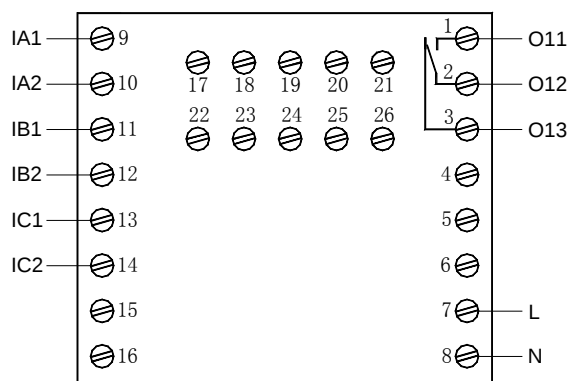
AMDPH-X/E001 系列保护器主单元接线端子图
