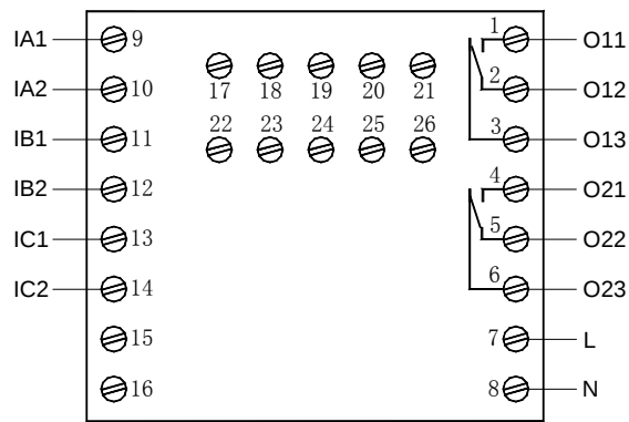
AMDPH-X/E002 系列保护器主单元接线端子图
