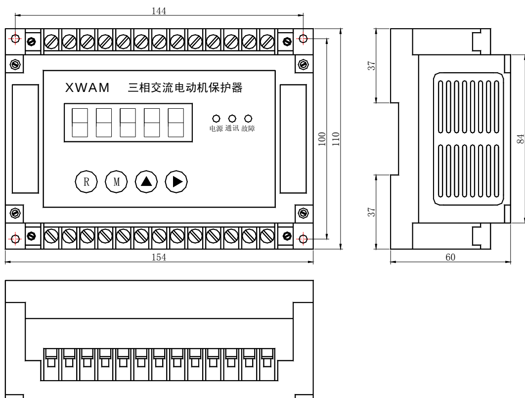
AMDG-X/F33□ 系列电动机保护器主单元外形及安装孔尺寸
