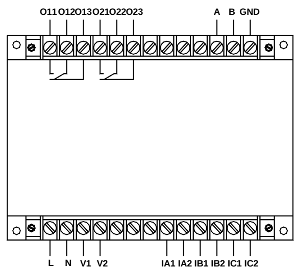
AMDG-X/F332 系列保护器主单元接线端子图
