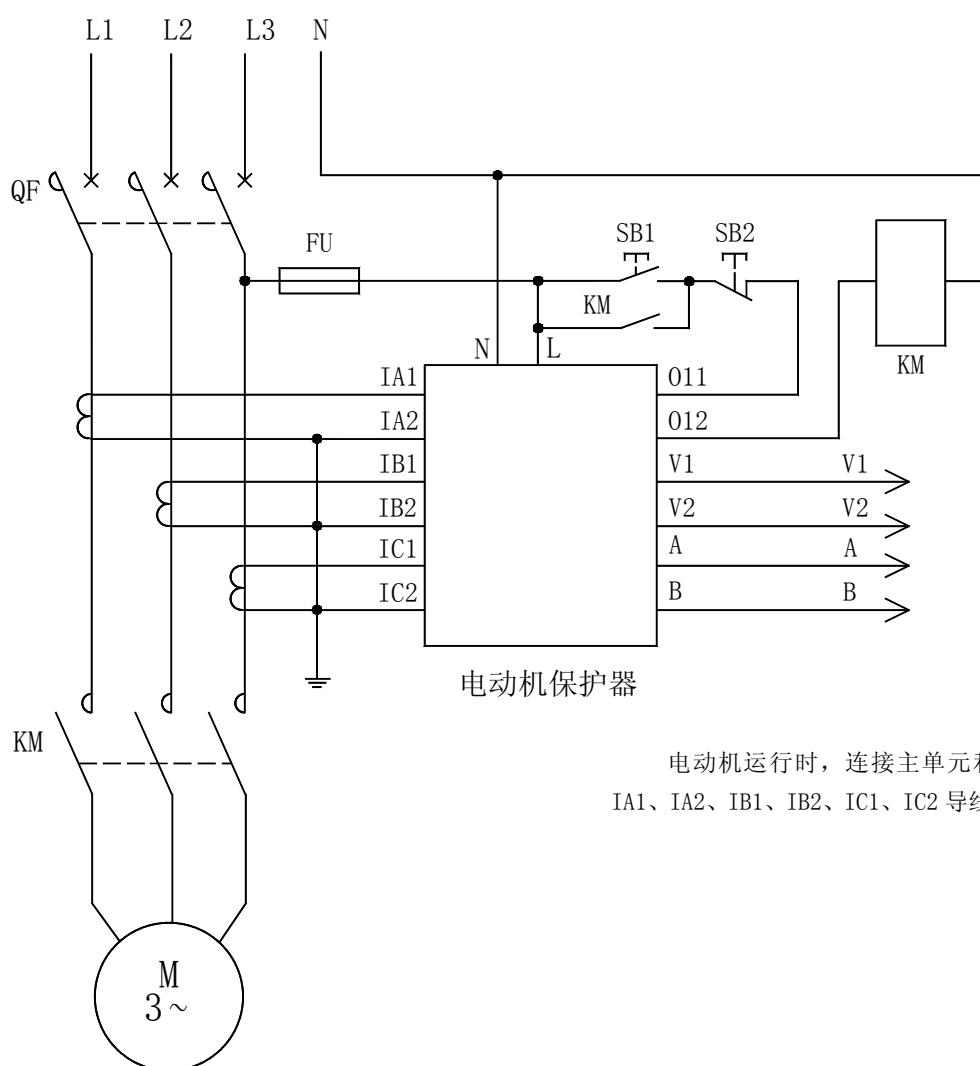
AMDG-X/F33□ 系列电动机保护器应用电气原理图
