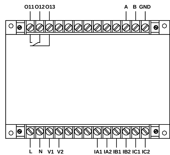
AMDG-X/F331 系列保护器主单元接线端子图
