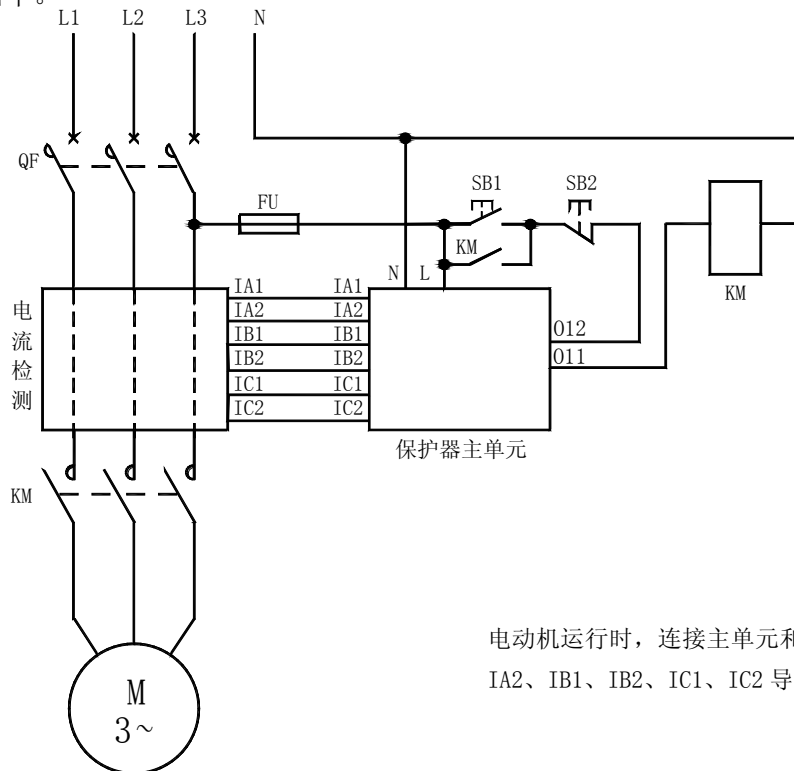
AMDS-□/A 系列电动机保护器应用电气原理图
