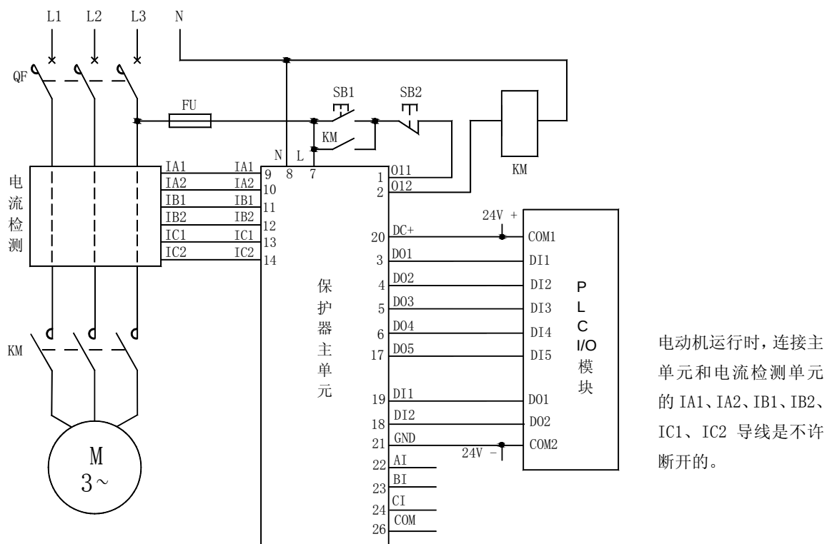
AMDP-□/C8 系列电动机保护器应用电气原理图
