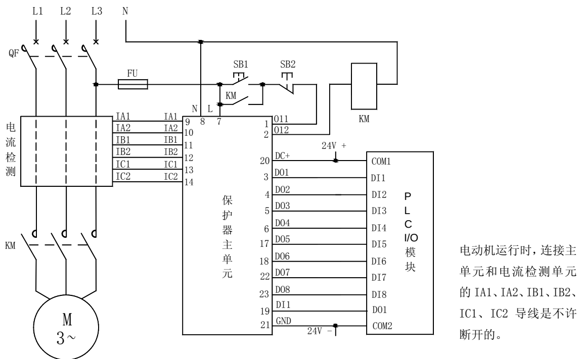
AMDP-□/C5 系列电动机保护器应用电气原理图
