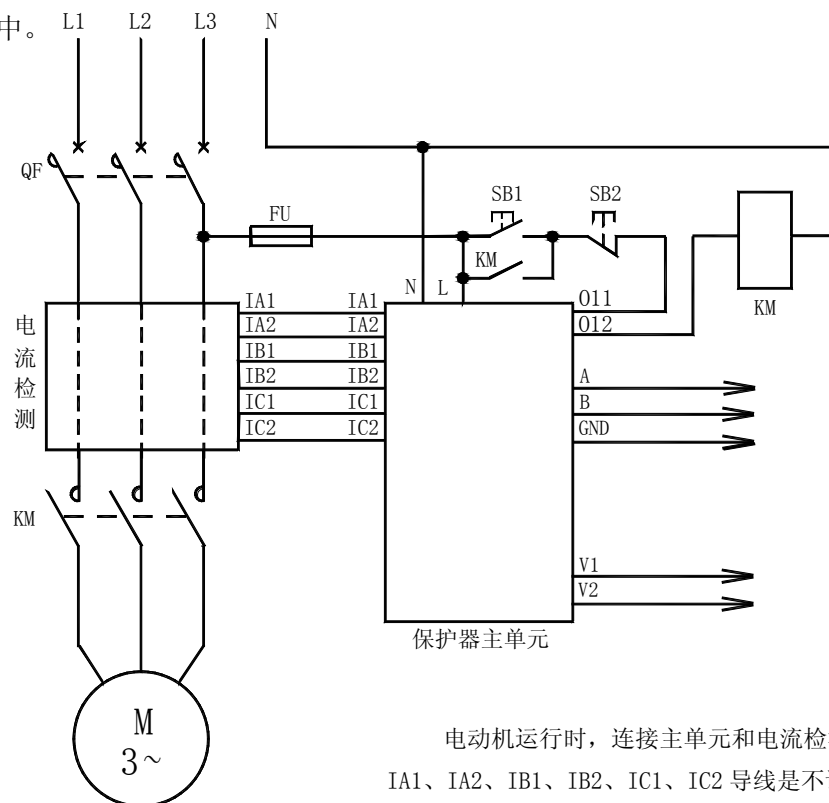
AMDG-□/D3 系列电动机保护器应用电气原理图
