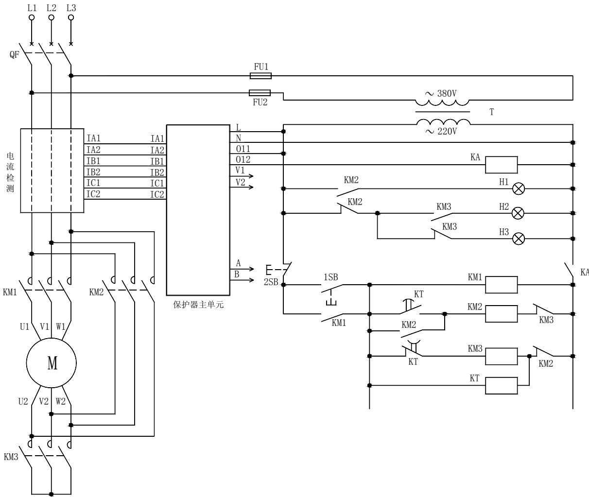
图 2 电动机保护器用于星/三角启动（检测线电流）电气原理图
