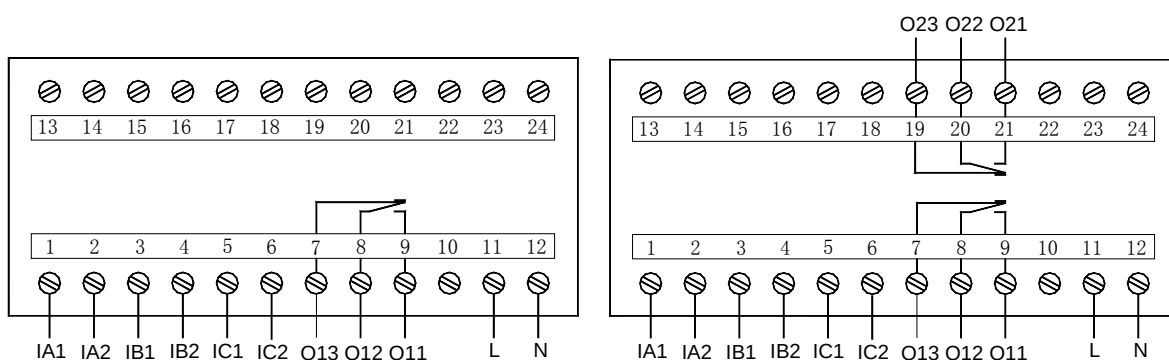
AMDP-□/B001 系列保护器主单元端子图
