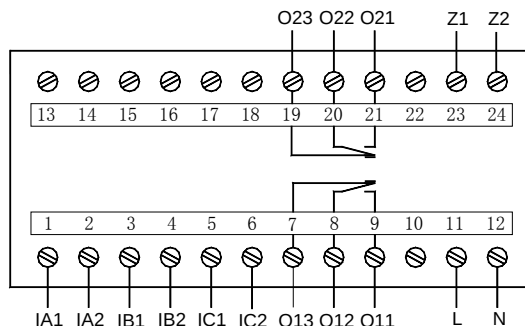
AMDP-□/B012 系列保护器主单元端子图
