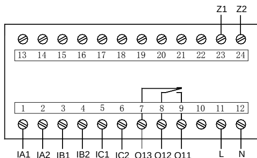
AMDP-□/B011 系列保护器主单元端子图
