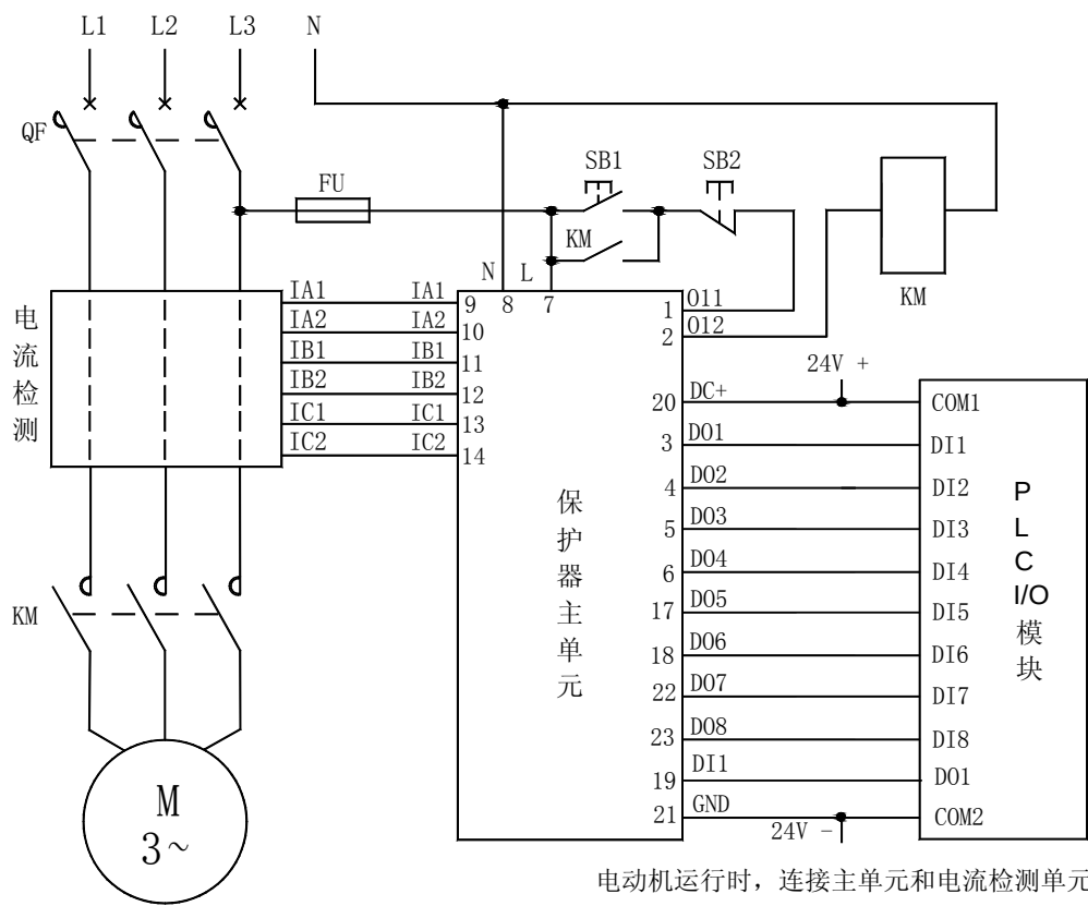
AMDP-□/C5 系列电动机保护器应用电气原理图
