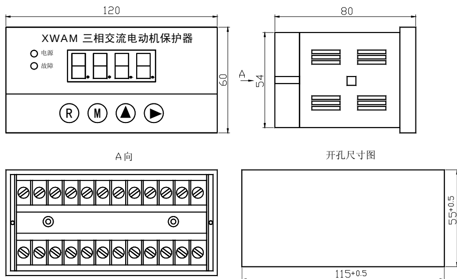
AMDP-□/□/□ 系列电动机保护器主单元外形及安装孔尺寸
