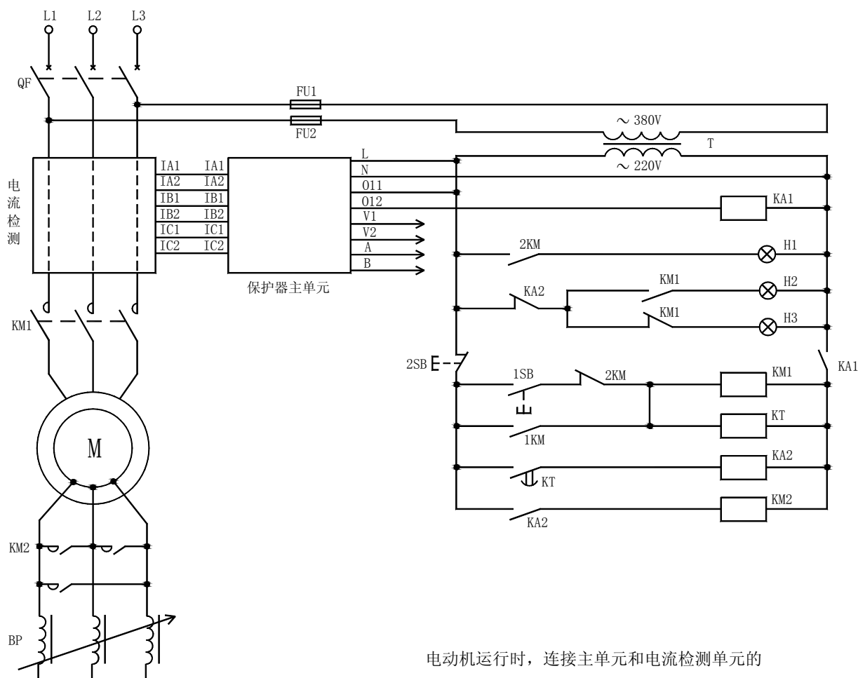
IA1、IA2、IB1、IB2、IC1、IC2 导线是不许断开的。
