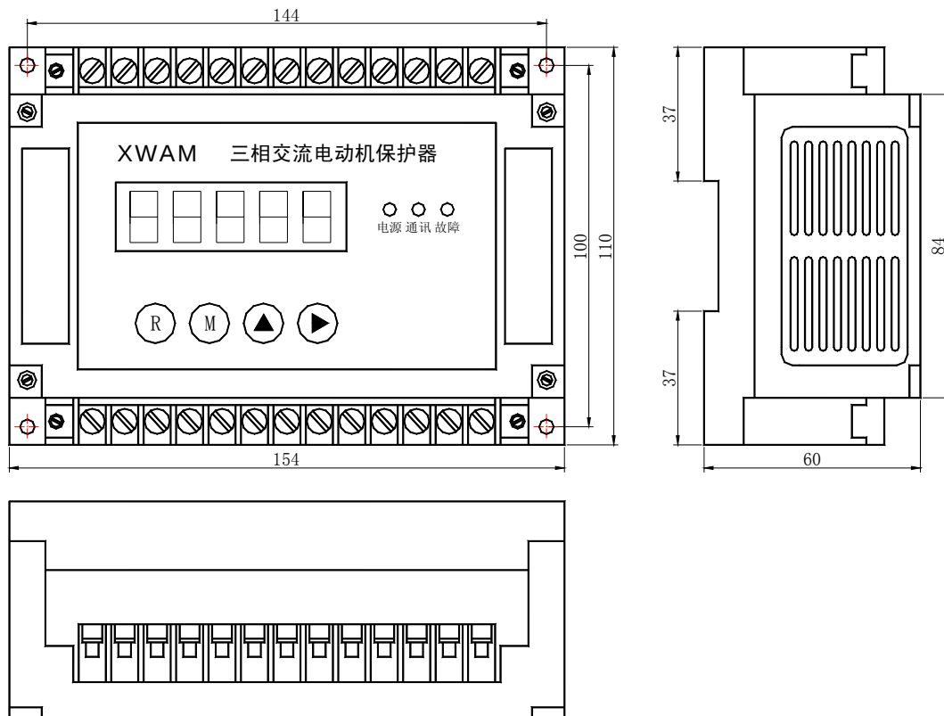
AMDG-□/D3 系列电动机保护器主单元外形及安装孔尺寸
